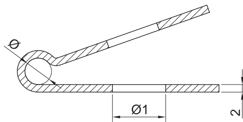
Corte A-A
